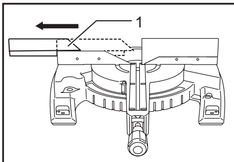
► 1. Sliding fence
