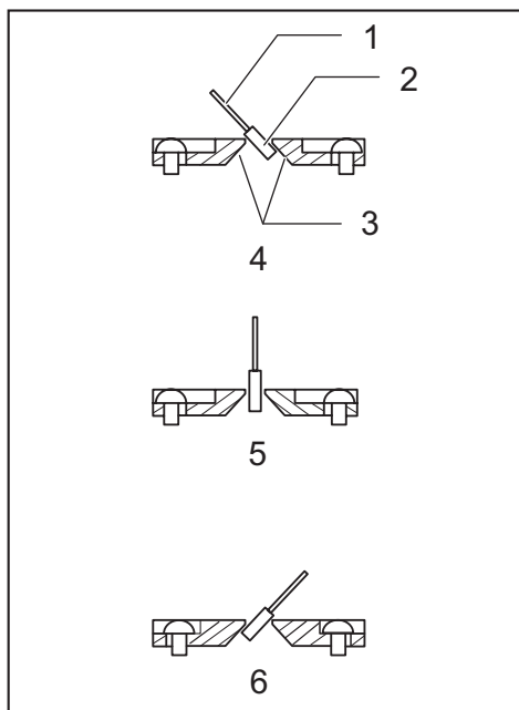
► 1. Lame 2. Dents de la lame 3. Plateau de découpe 4. Coupe en biseau sur la gauche 5. Coupe rectiligne 6. Coupe en biseau sur la droite
