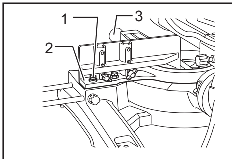
► 1. Tornillo hexagonal 2. Guía lateral 3. Empuñadura
