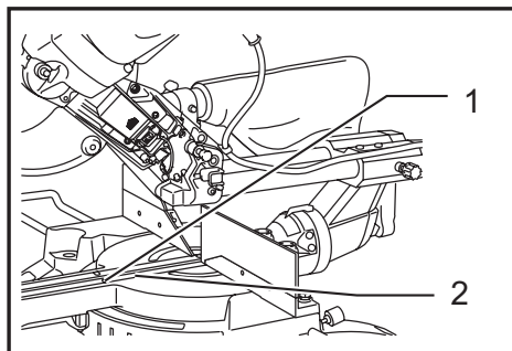
► 1. Screw 2. Kerf board
