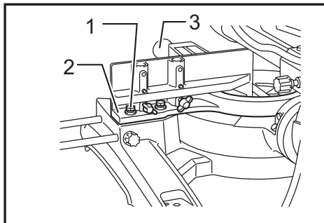
► 1. Hex bolt 2. Guide fence 3. Grip
