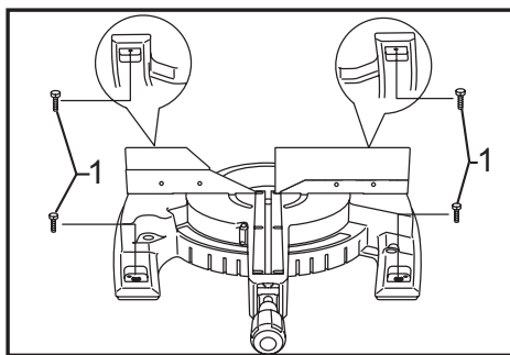
► 1. Boulons
